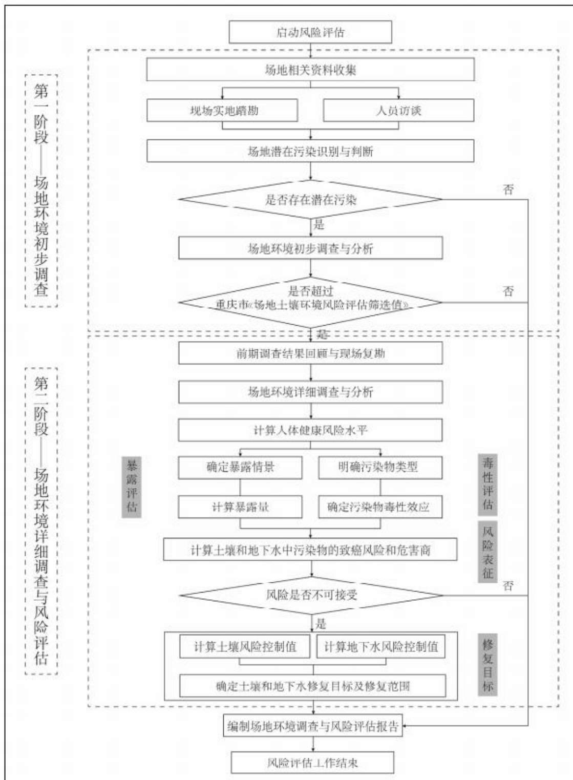
图 1.6-1 场地环境调查与风险评估工作程序图
