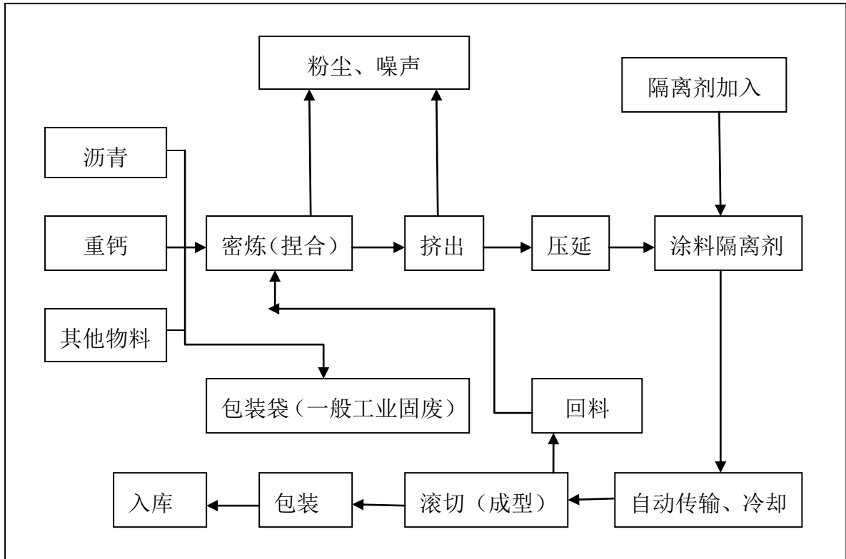
图 2.2-10 沥青阻尼板生产工艺流程图
