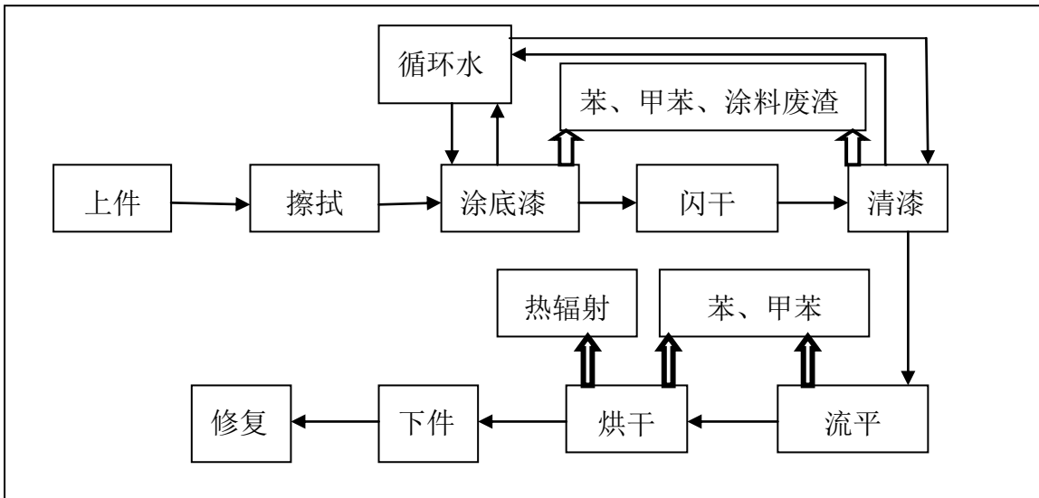
图 2.2-8 护板装饰件生产工艺流程图
