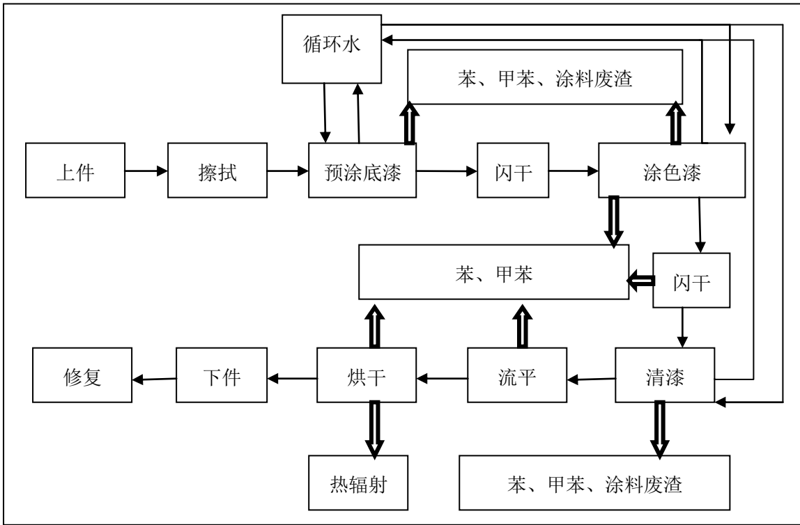
图 2.2-7 保险杠生产工艺流程图
